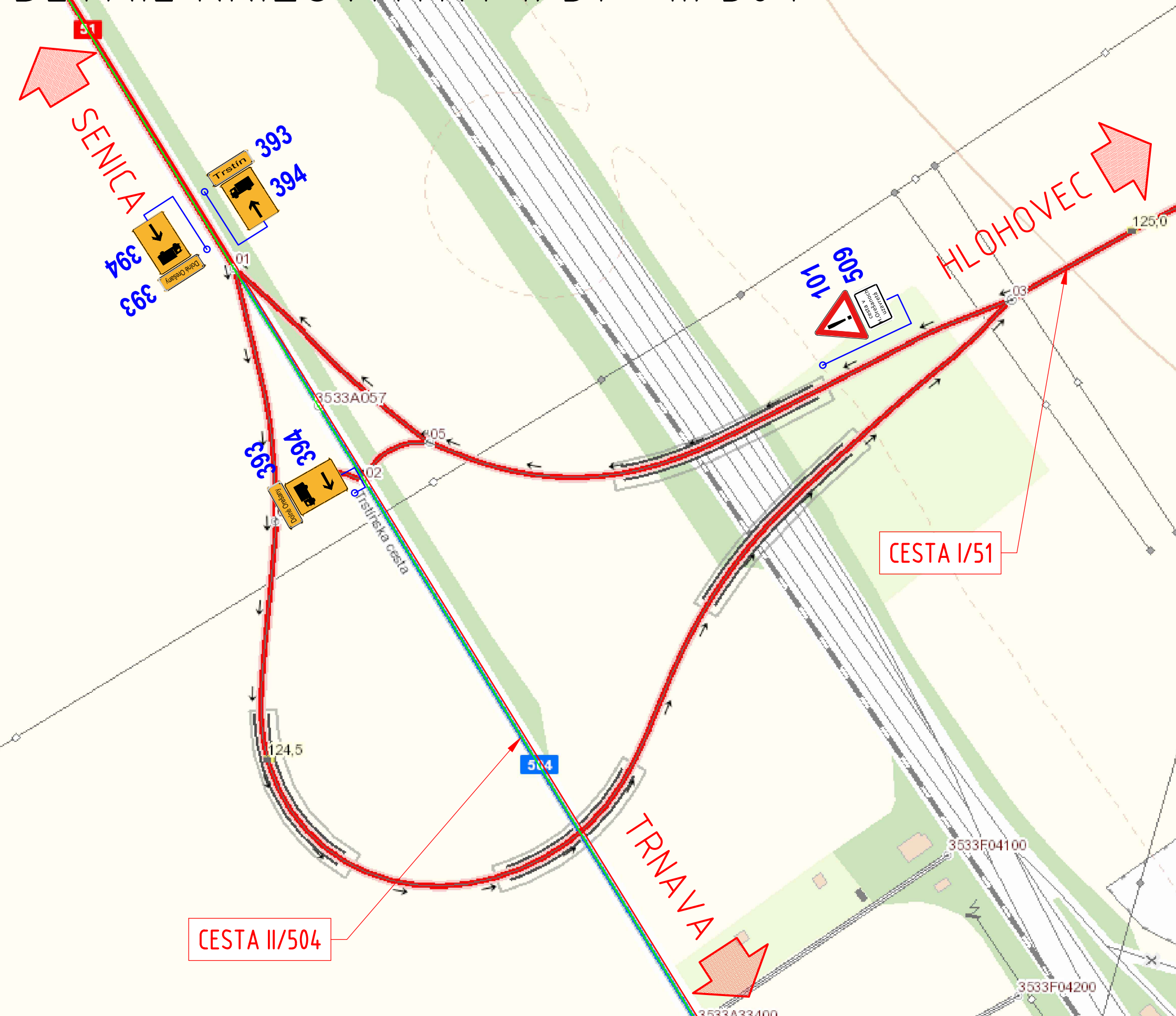
DETAIL KRIŽOVATKY I/51 – II/504
