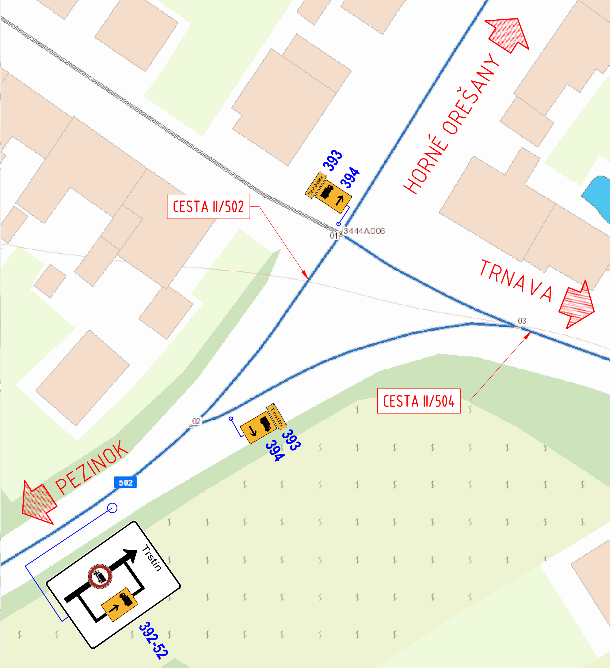
DETAIL KRIŽOVATKY II/502 – II/504
