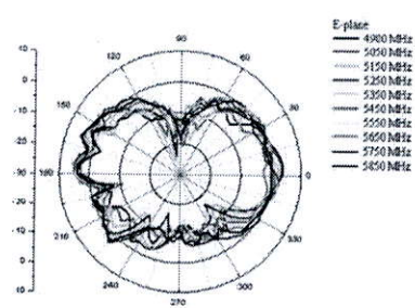
5GHz E-Plane
