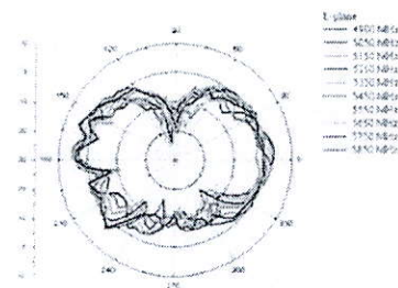
5GHz E-Plane
